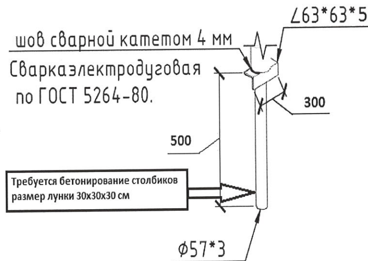
Рис. 2. Монтаж на металлические закладные
